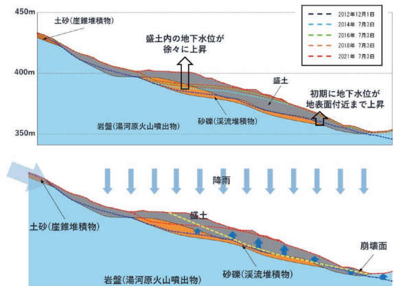
図3-2 盛土完成後に、地表水である水が盛土内に浸透し、地下水位が上昇。さらに降雨によって水位が上がることで崩壊が起こることを解析で明らかにした。
