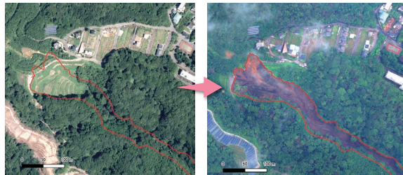
図3-1 崩壊前後の地表面と地下水位の変化。盛土を埋めるように盛土が施工されたが、降雨により後に崩壊。地下水が原因だと判明していたが、記録やデータは残っていない状態だった。
