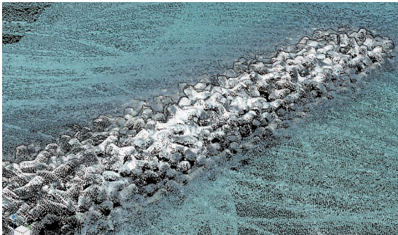
図4-2 現地の計測データから作成された消波堤の3次元データ(点群)
